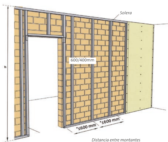
Distancia entre montantes
